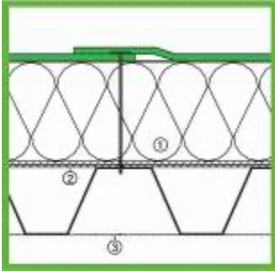
Mekanik tespit metodu 1) Isı yalıtımı katmanı 2) Alt yapı katmanları 3) Trapezoidal metal çatı levhası 4) KÖSTER TPO Pro Sentetik Örtü (yeşil katman)
